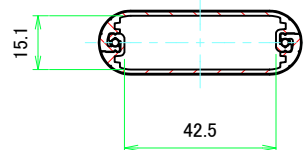
A-A (1:1.5)
